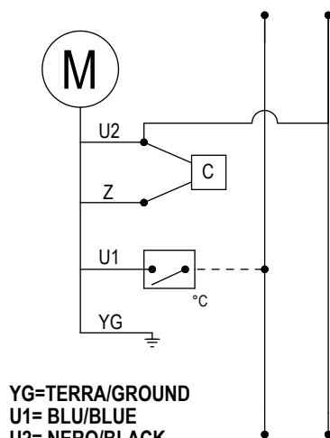
COLLEGAMENTO ELETTRICO 230V MON. AC 230V AC MON. ELECTRIC WIRING
