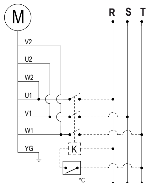
COLLEGAMENTO ELETTRICO 230V AC TRIF. 230V AC THREEPHASE ELECTRIC WIRING
